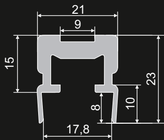
Profil łączący do rury 20x20 Профиль соединительный для трубы 20x20 nr 037 012 05
