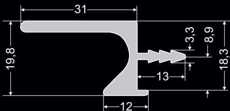
Uchwyt do szafek dolnych Ручка-планка для нижних шкафчиков
